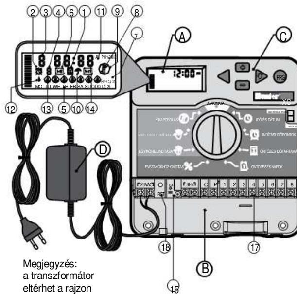
Beltéri típus
