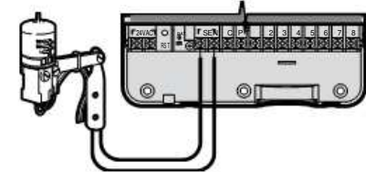
Mini-Clik esőérzékelő
