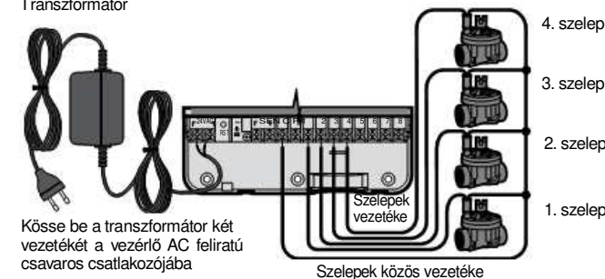
Transzformátor
