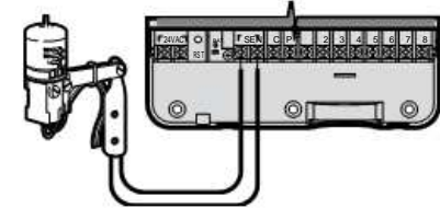
Mini-Clik esőérzékelő
